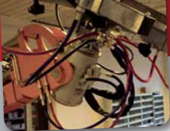
Det multifunktionelle, hydrauliske drejehoved.
